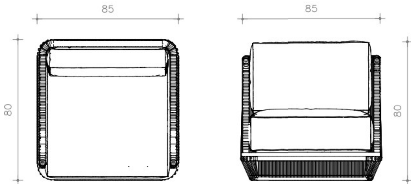
VISTA SUPERIOR
